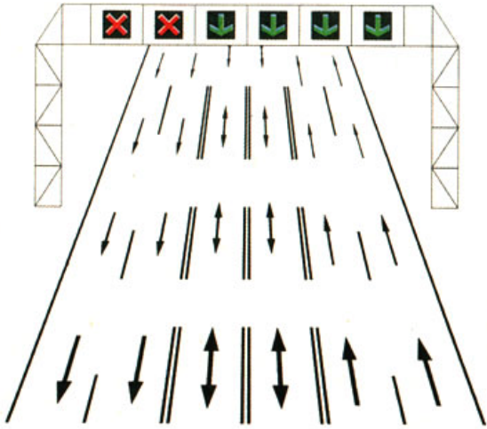
Dispozitive luminoase pentru dirijarea circulatiei pe benzi reversibile
